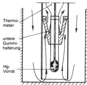
Strömung des Wassers beim Füllen des Gefäßes (Prinzip)
